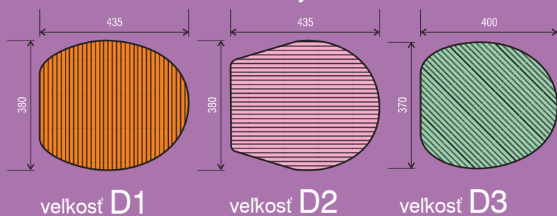
Velkosti a tvary dosiek
